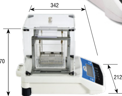
Dimensiones (mm)
